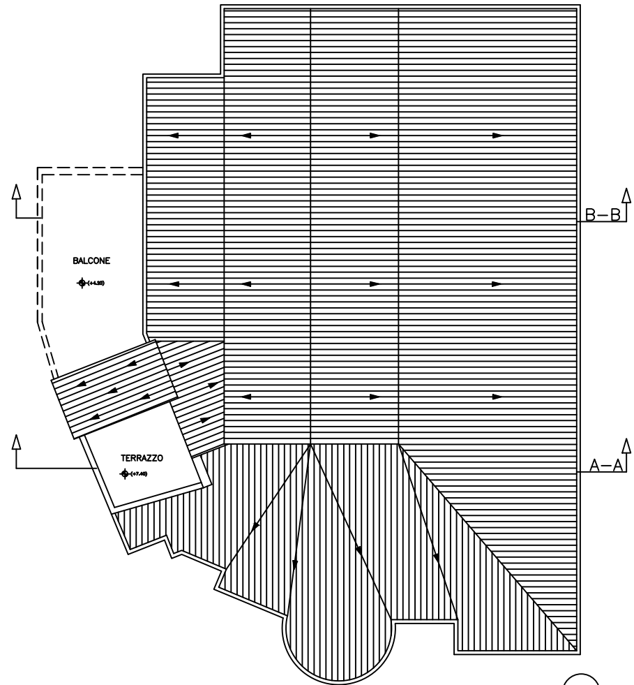
PIANTA COPERTURA SCALA 1:100
