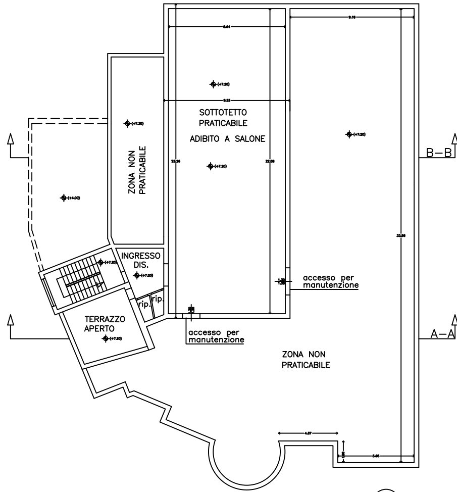
PIANTA SOTTOTETTO DELL'INTERO PIANO ZONA ABITABILE SCALA 1:100
