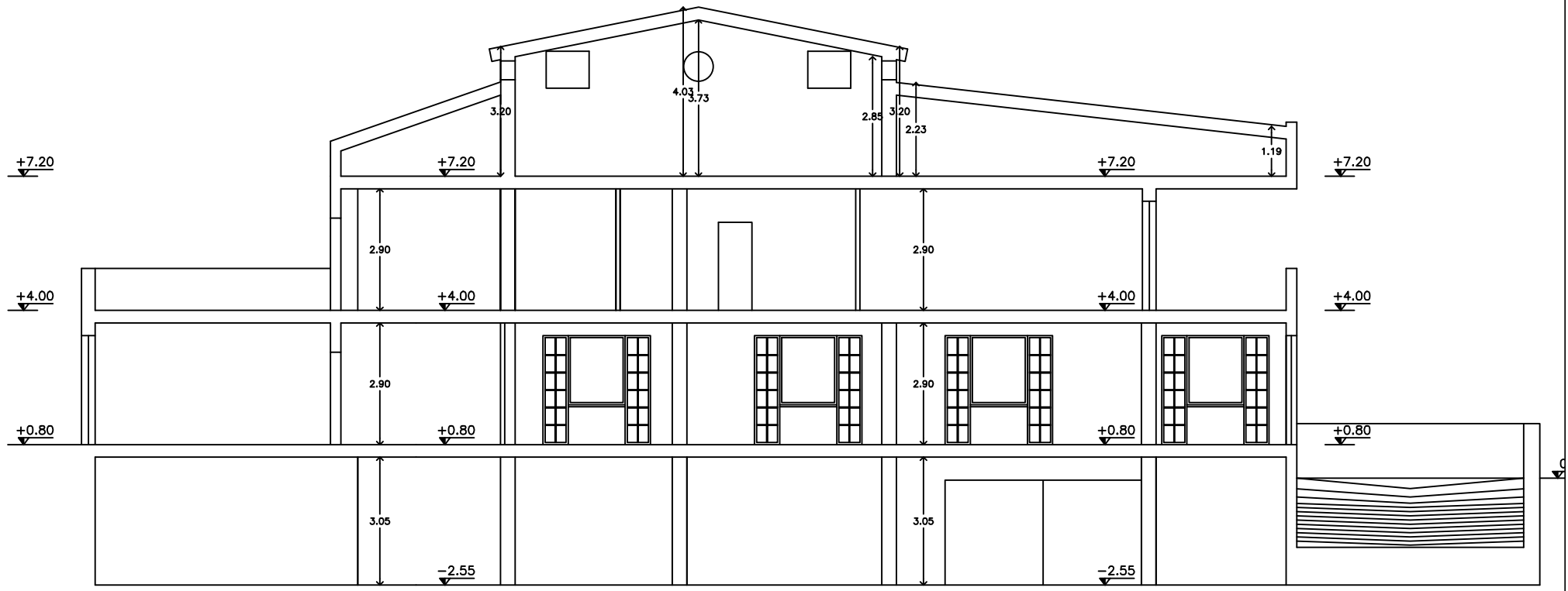
SEZIONE B-B Scala 1:100
