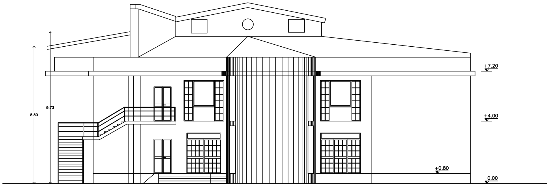
PROSPETTO Scala 1:100
